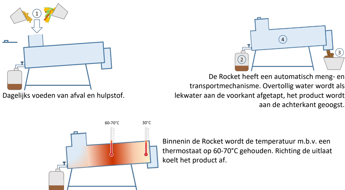
Figuur 17. Schematische weergave van het gebruik van de Rocket (afbeelding: IB). Het deksel wordt eraf gehaald. Verkleind afval en hulpstof ① worden bovenin gevoed. Lekwater wordt wanneer nodig vooraan afgetapt ②, het product wordt aan de achterkant geoogst ③. Het transport van het materiaal in de Rocket gebeurt automatisch ④. Het product moet nog narijpen.
