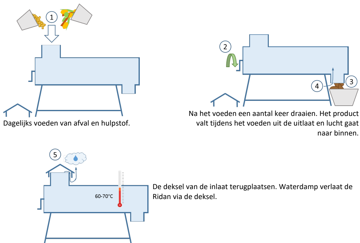
Figuur 15. Schematische weergave van het gebruik van de Ridan (afbeelding: IB). Het deksel wordt eraf gehaald. Verkleind afval en hulpstof ① worden bovenin gevoed. Na het voeren het roerwerk ② minimaal 6 keer draaien. Het product valt er dan via de uitlaat uit ③ en verse lucht ④ gaat er via de uitlaat in. Het product moet nog circa 3 maanden nagecomposteerd worden. Bij correct gebruik loopt de temperatuur hoog op. Waterdamp verlaat de Ridan via de deksel ⑤.
